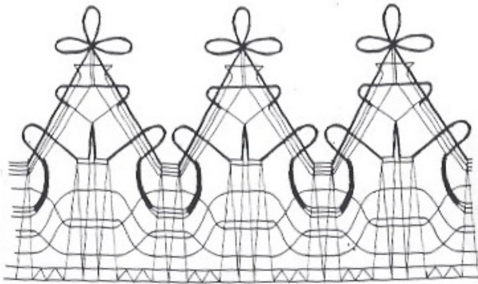
Werkschema
